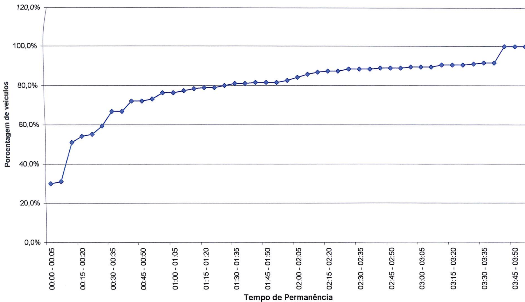
Gráfico C10.3 - Tempo de Permanência (Acumulado) C 10 - Centro de Convenções do Othon
