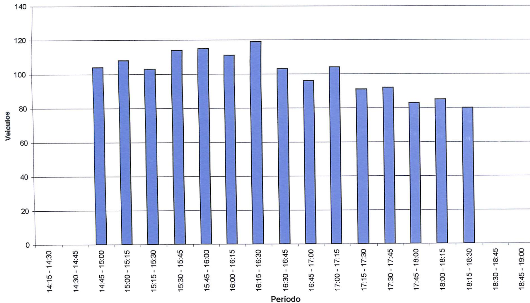
Gráfico C10.1 - Ocupação do Estacionamento C 10 - Centro de Convenções do Othon
