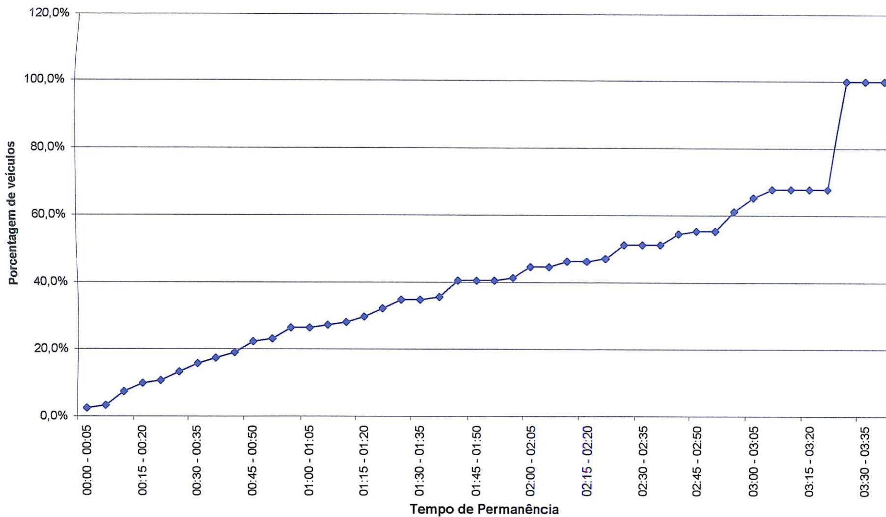
Gráfico C15.3 - Tempo de Permanência (Acumulado) C 15 - Fiesta Convention Center
