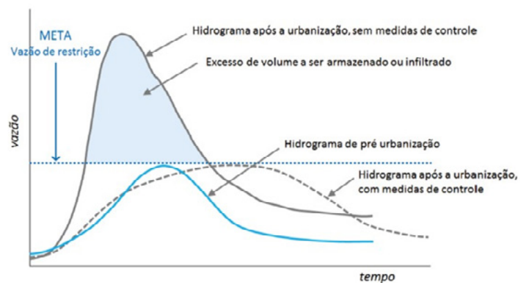
Figura 29 – Representação dos hidrogramas e vazão pluvial nas fases de pré e pós-urbanização, com indicação de meta de restrição
