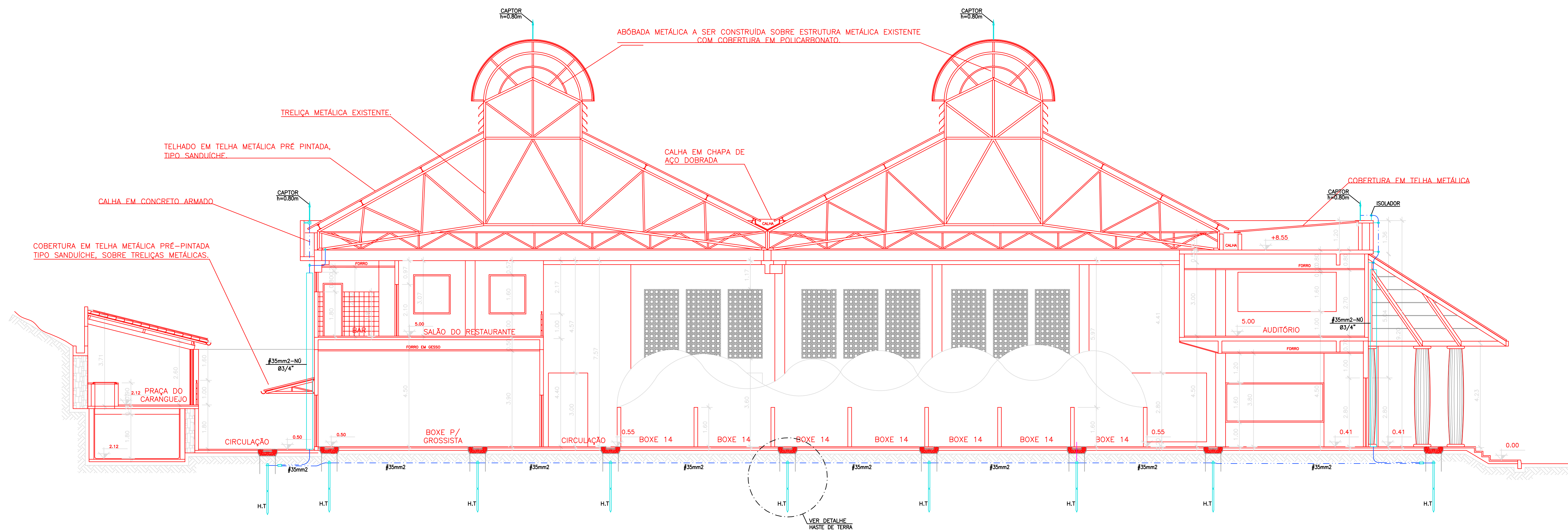
CORTE DD
