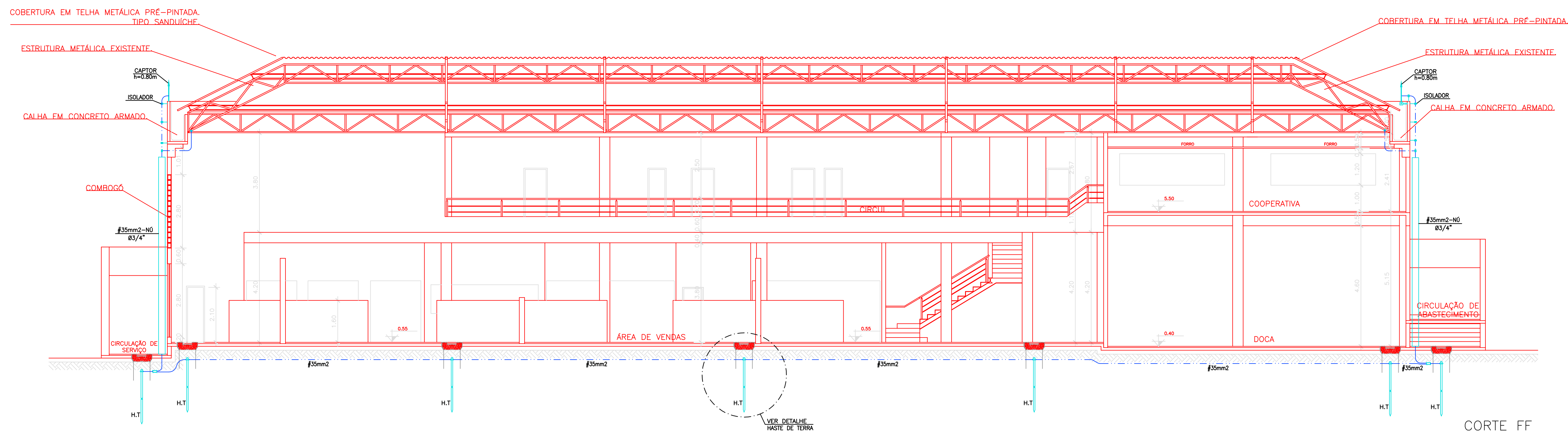
CORTE FF
