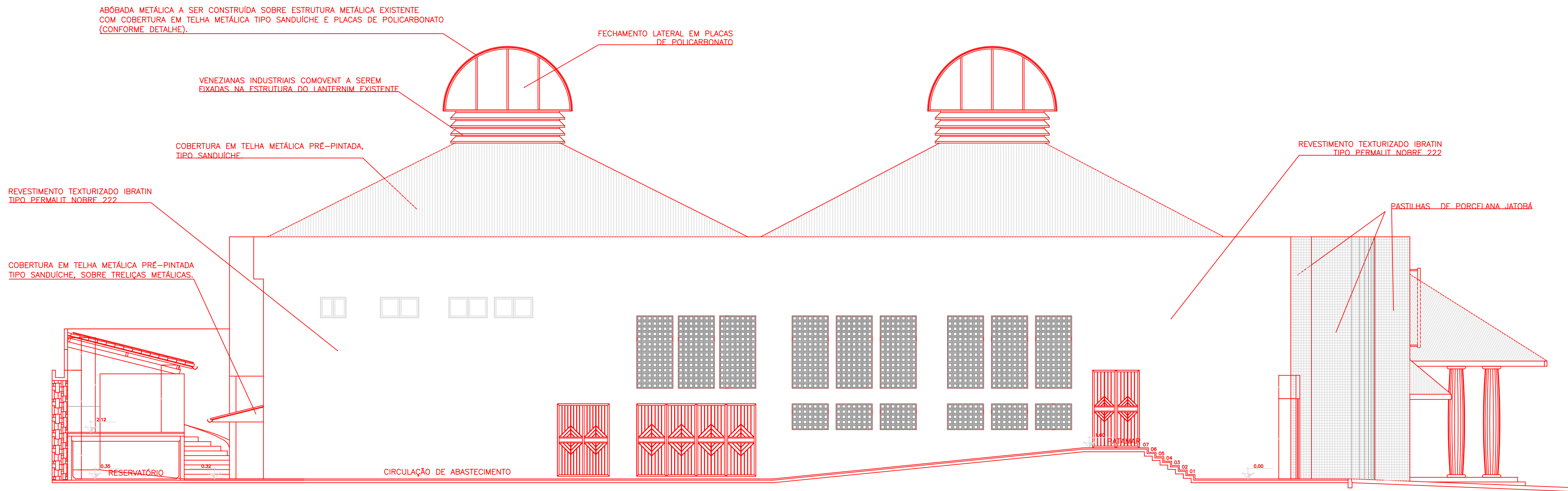
FACHADA 03
