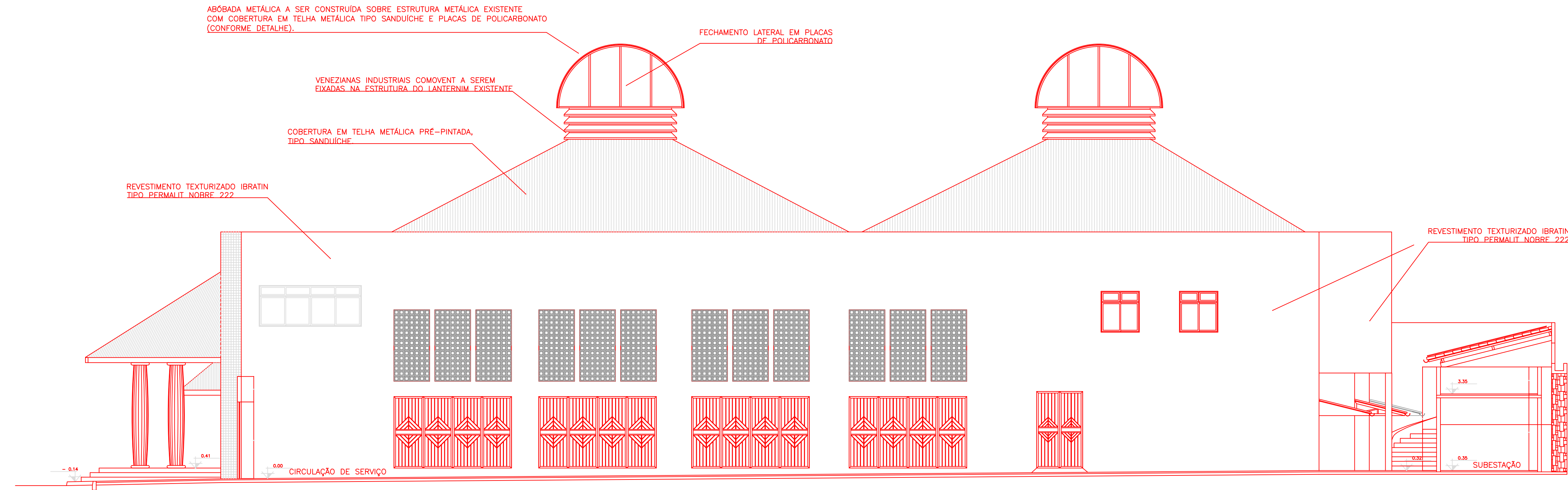
FACHADA 04
