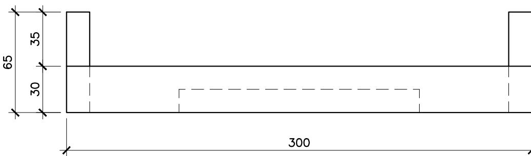
VISTA G-G ESC. 1:25
