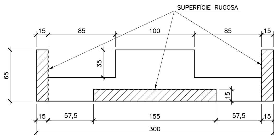
CORTE M-M ESC. 1:25
