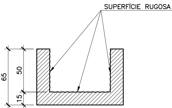
CORTE D-D ESC. 1:25
