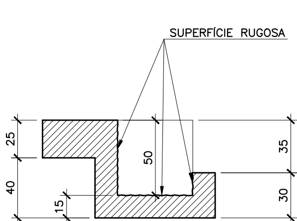
CORTE H-H ESC. 1:25
