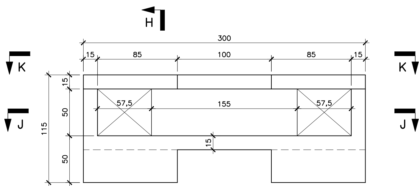
VPM4 - PLANTA (1x) ESC. 1:25
