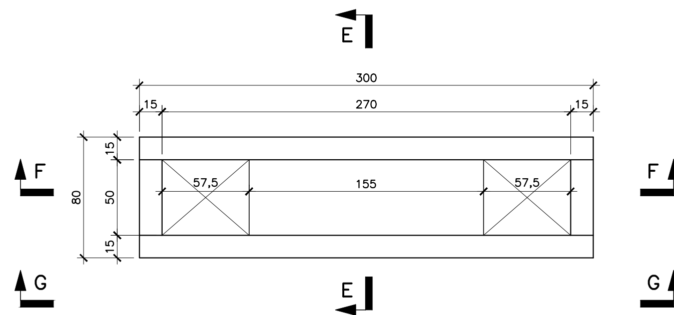
VPM3 - PLANTA (4x) ESC. 1:25
