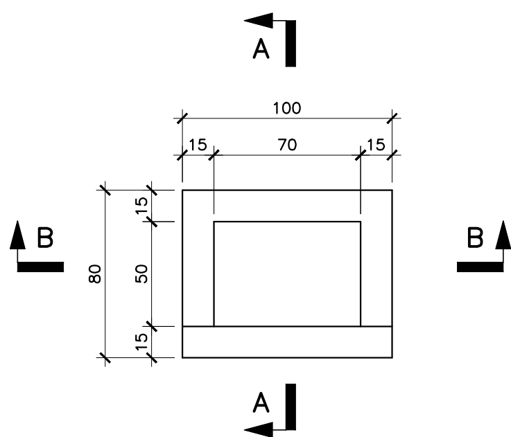
VPM1 - PLANTA (1x) ESC. 1:25
