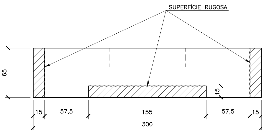
CORTE J-J ESC. 1:25
