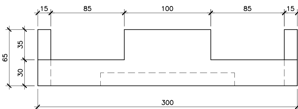
VISTA K-K ESC. 1:25
