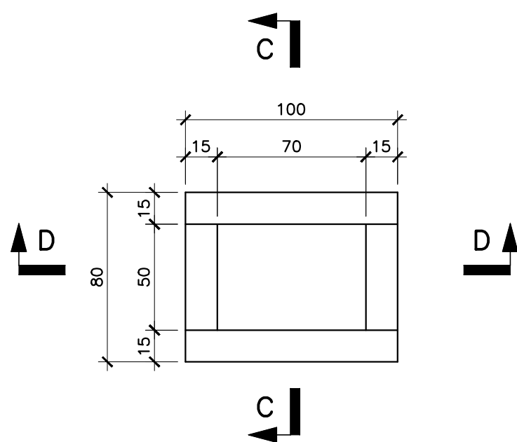
VPM2 - PLANTA (1x) ESC. 1:25
