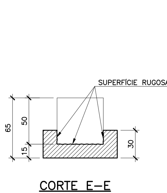
CORTE E-E ESC. 1:25
