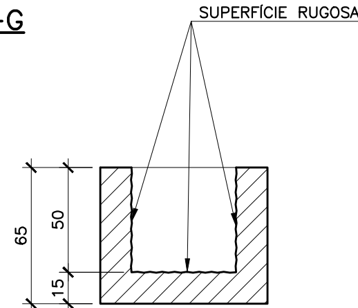
CORTE L-L ESC. 1:25
