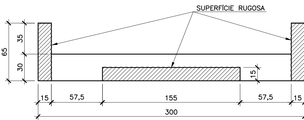
CORTE F-F ESC. 1:25
