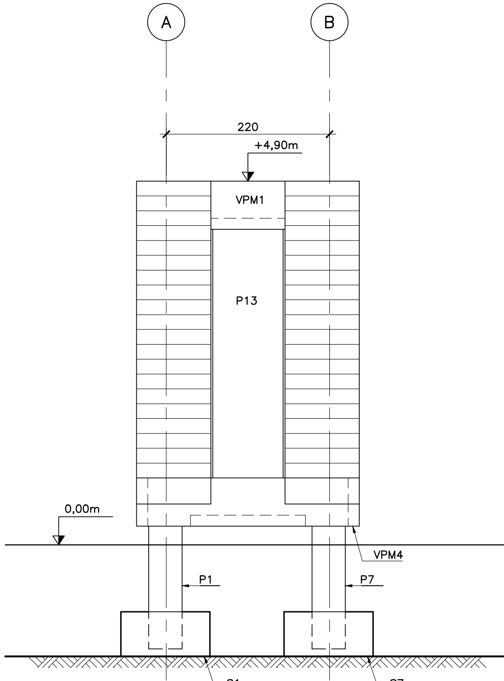
VISTA D-D ESC.1:50
