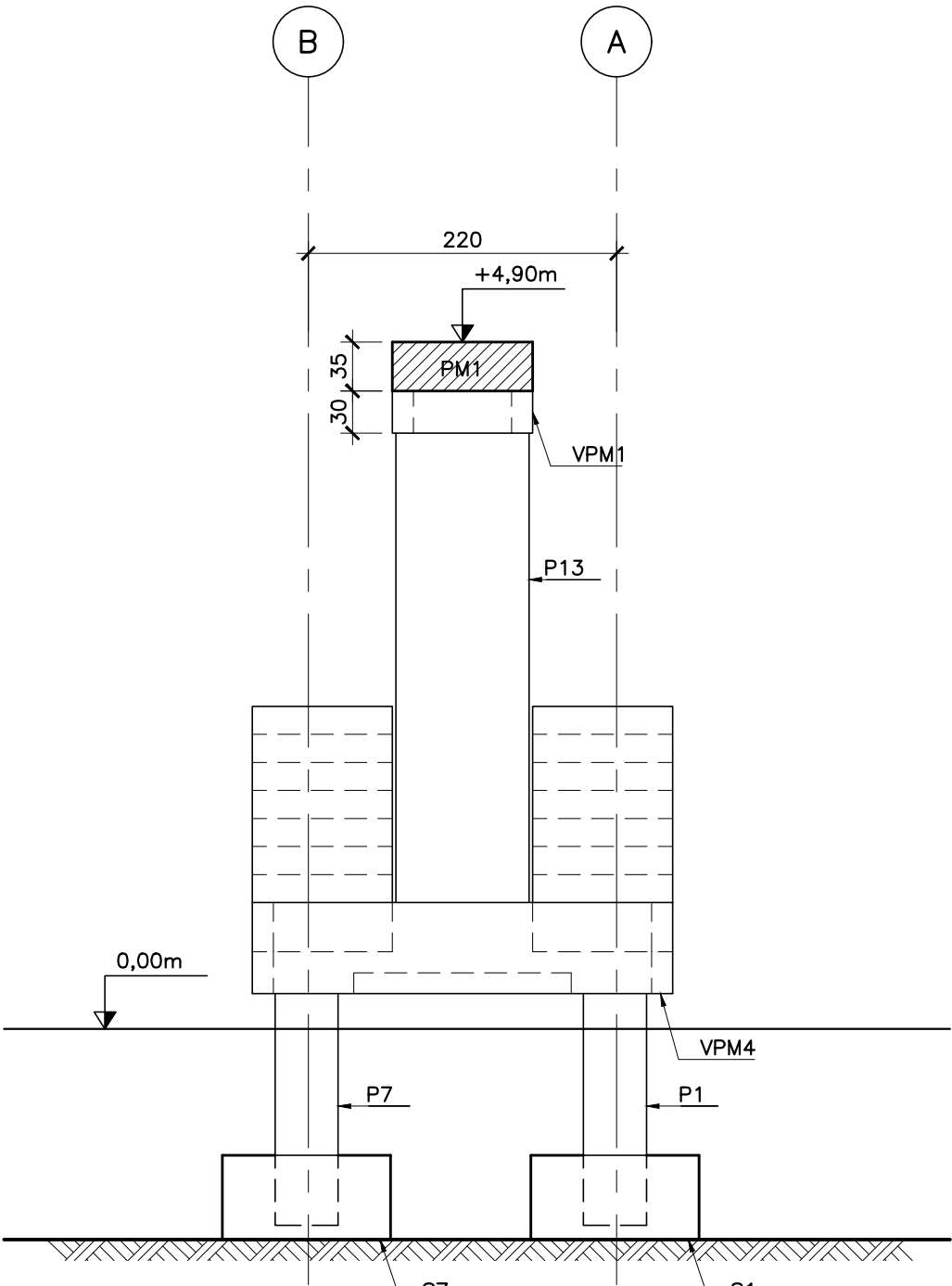
CORTE C-C ESC.1:50
