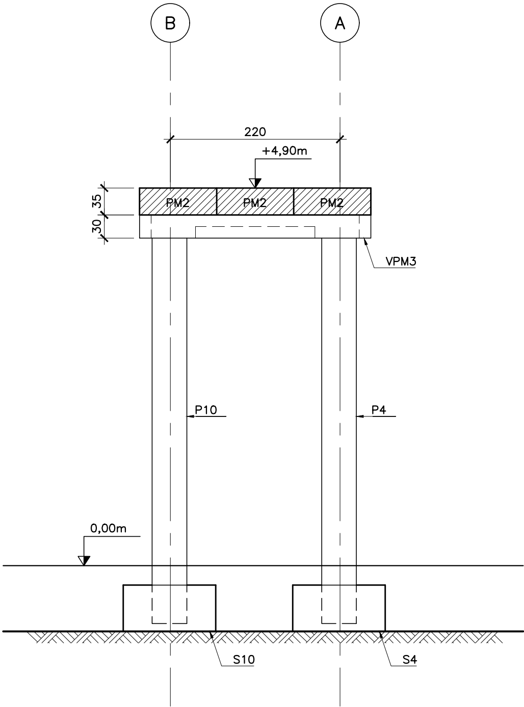
CORTE B-B ESC.1:50
