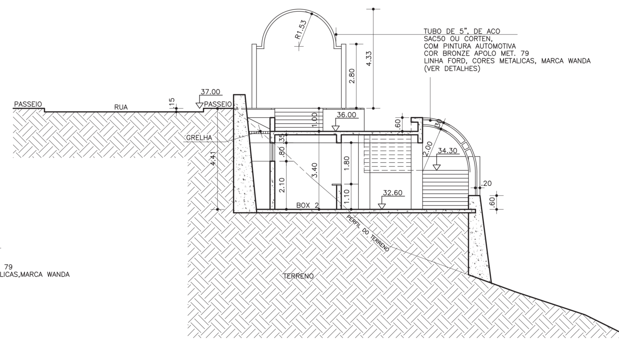
CORTE CC
