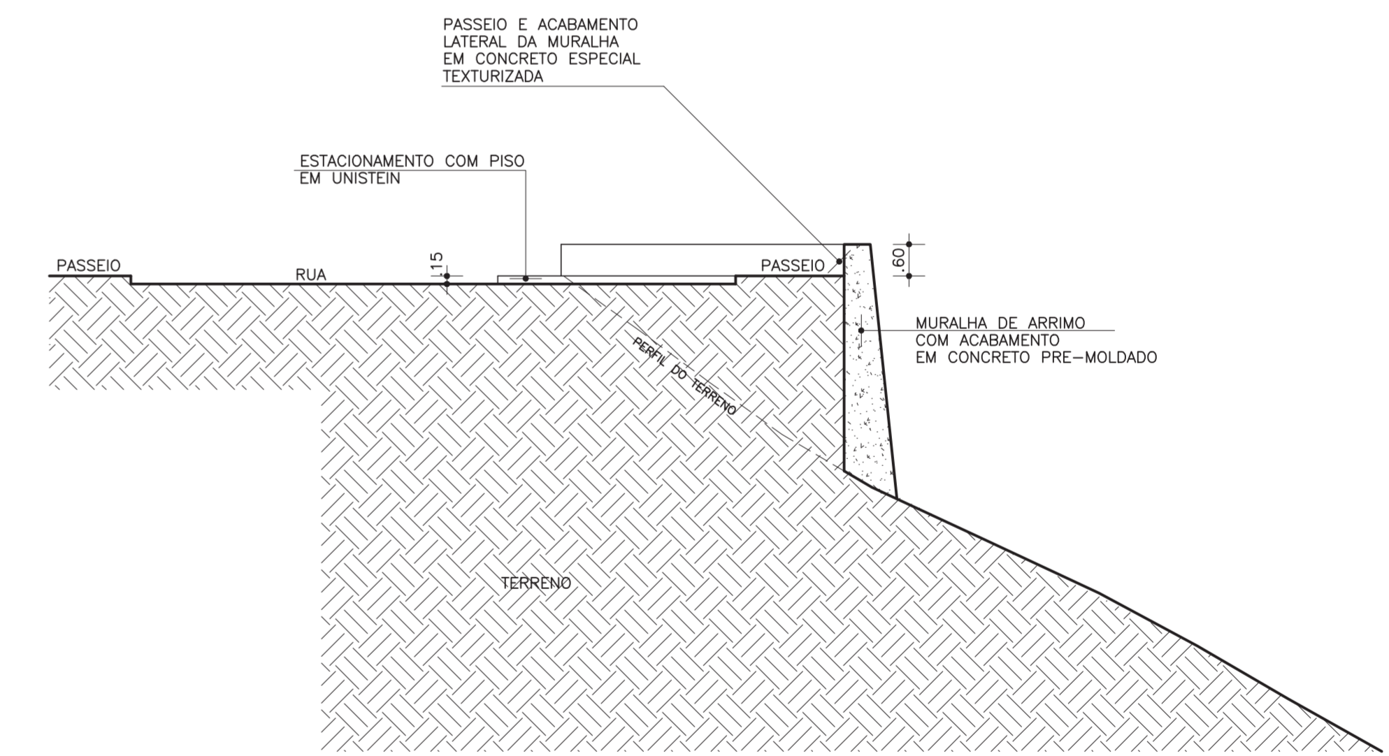
CORTE DD
