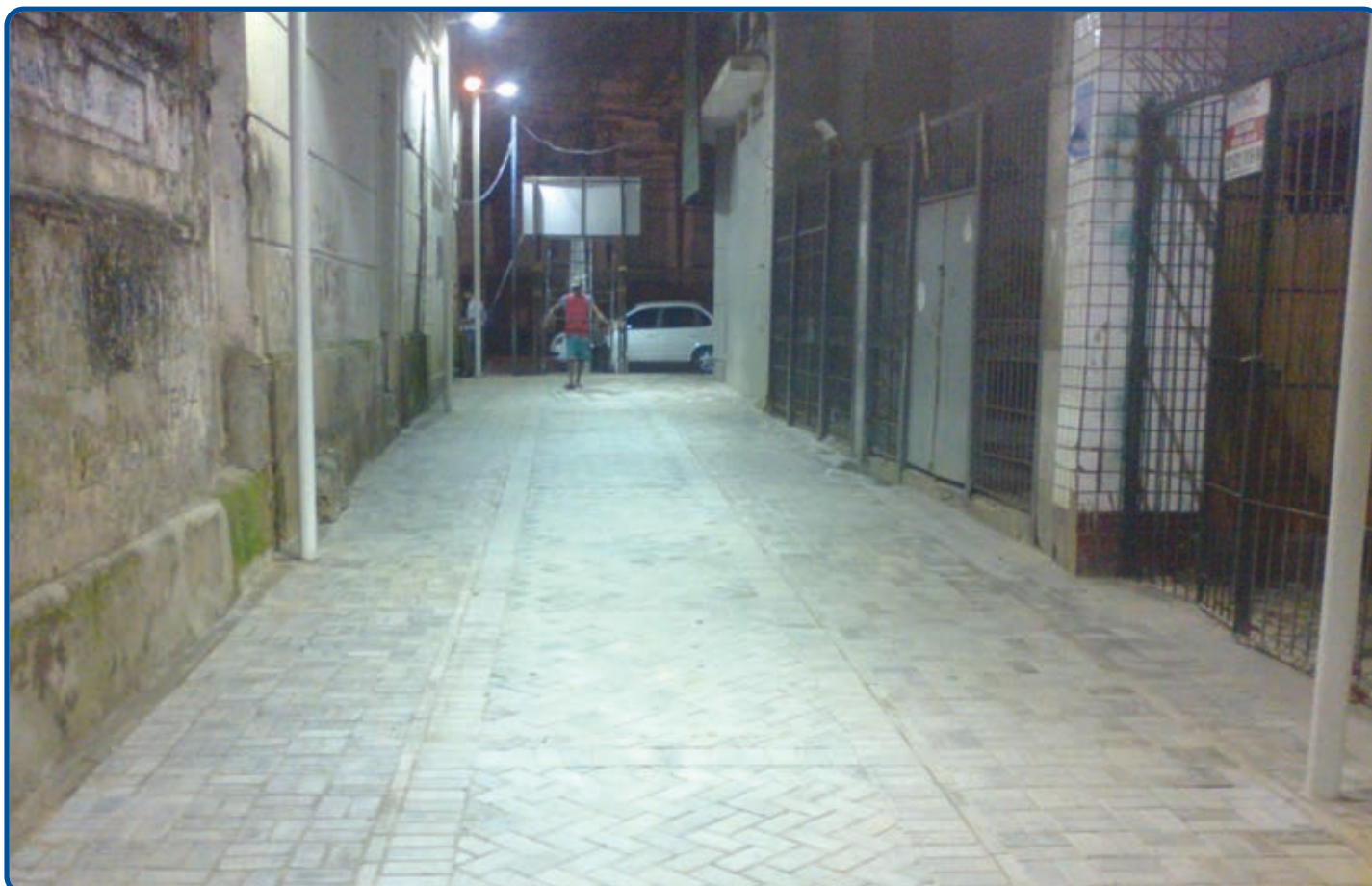
No Beco do Mucambinho já foi aplicado o novo piso intertravado, em substituição às pedras portuguesas, e limpeza das caixas de drenagem e esgoto
